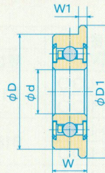
【フランジ・シール形】
