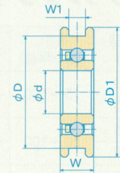
【両フランジ形】
